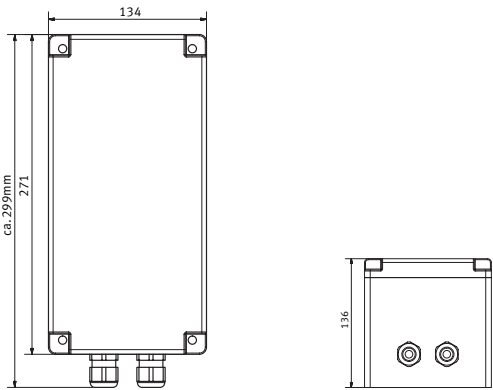
Abmessungen des OPTIME Ex Gateway
