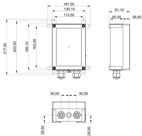
Abmessungen des OPTIME Gateway
